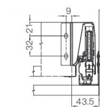
背板安装尺寸 Back installation dimensions 单位 unit:mm
