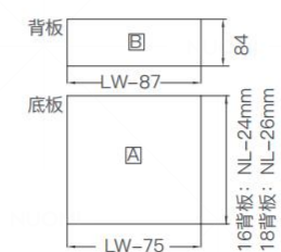
2. 用于 16/18mm 密度板的 裁切尺寸 Cutting dim. for 16/18mm chipboard
