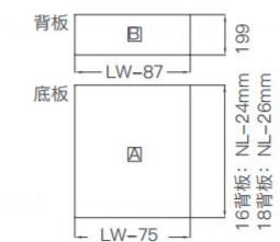
2. 用于 16/18mm 密度板的 裁切尺寸 Cutting dim. for 16/18mm chipboard
