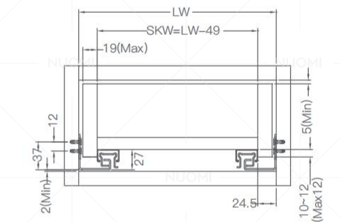
滑轨安装孔位 Hole position
