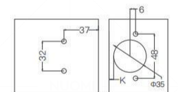
Hole Size 钻孔尺寸
