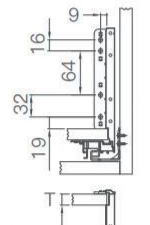
背板安装尺寸 Back installation dimensions 单位 unit:mm
