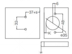
Hole Size 钻孔尺寸
