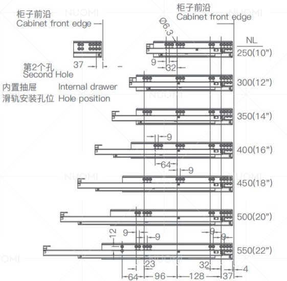
滑轨安装孔位 Hole position
