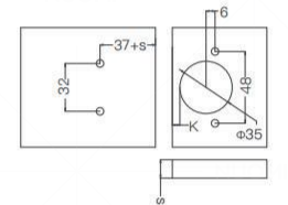
Hole Size 钻孔尺寸
