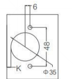
Hole Size 钻孔尺寸
