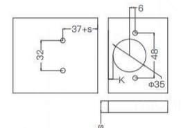
Hole Size 钻孔尺寸
