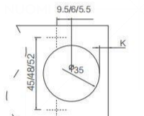
Hole Size 钻孔尺寸
