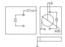
Hole Size 钻孔尺寸
