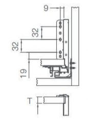
背板安装尺寸 Back installation dimensions 单位 unit:mm
