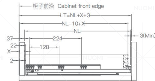
内置抽屉 Internal drawer
